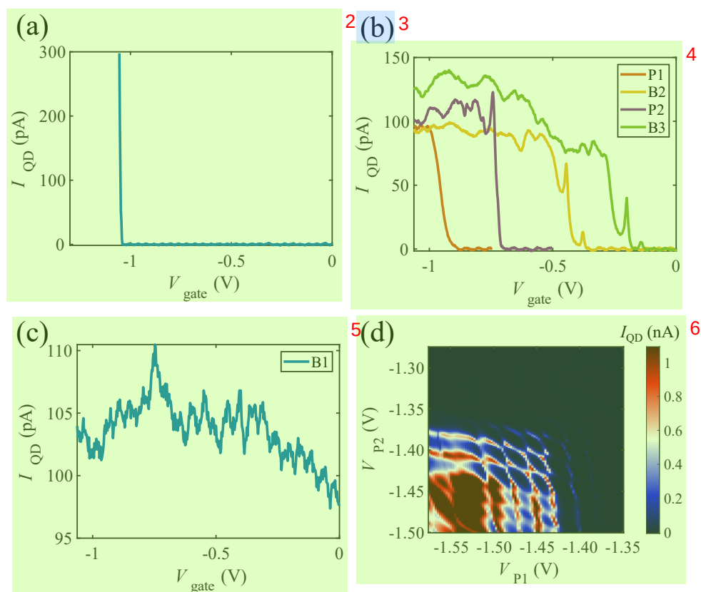
图 3.10 (a) 量子点开启时的 I - V 曲线，开启的电压约为 -1 V。(b) 量子点栅极夹断时的 I - V 曲线，每根电极的调节能力不同，夹断的电压也有所不同，但它们都具有独立调控沟道打开与夹断的能力。(c) 量子点的栅极不能独立地夹断量子点沟道，该电极的性能不符合预期。造成这种现象的原因可能是栅极没有落入沟道之中或者在栅极扇出的过程中发生了断路。(d) 呈现出蜂窝状的双量子点输运相图。
