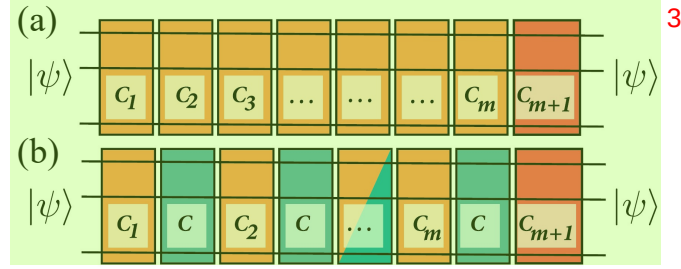
图 2.7 随机基准测试中的两种实验序列 (a) 标准基准测试序列示意图。 C_1-C_m 是随机从 Clifford 门中选取的 m 个门操作。执行最后的 C_{m+1} (红色) 以使总序列等于恒等操作。(b) 交错基准测试序列的示意图， C (绿色) 与从 Clifford 中选择的随机门 C_i (橙色) 交错，执行最后的门 C_{m+1} (红色) 以使总序列等于恒等操作。图源自 [143] 。
