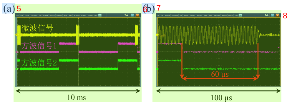
图 3.17 (a-b) 示波器测得微波信号与方波信号在同步触发条件下仍存在约 60\ \mu\text{s} 的相对延迟。(b) 为 (a) 的放大图，可以看出经过同步触发之后的微波信号与方波信号仍存在约 60\ \mu\text{s} 的相对延迟
