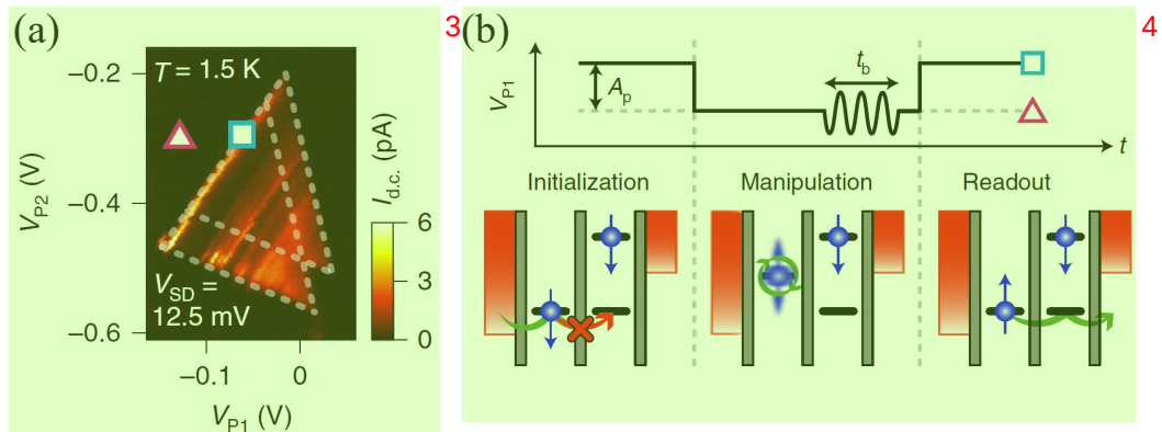
图 2.3 (a) 测量到的一对自旋阻塞偏置三角形。蓝色方块与粉色三角分别标示量子比特的初始化/读出位置以及操控位置。(b) 自旋操控循环的示意图，以及与之对应的脉冲时序方案。图源自 [128] 。
