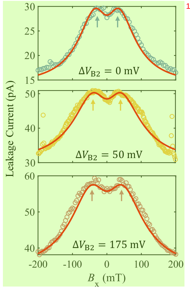
图 4.11 不同点间隧穿下的面外方向的漏电流磁谱，随着 \Delta V_{B2} 逐渐减小，点间隧穿被逐渐打开，同时自旋轨道耦合强度也被电压调控。
