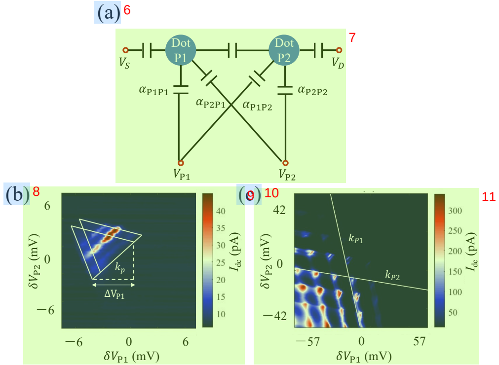
图 4.12 (a) 双量子点的等效电路图。柱塞电极 (P1 和 P2)、源极和漏极, 以及量子点本身和量子点之间的耦合, 都可以建模为电容耦合。 12 (b) 源漏偏压为 1 mV。在 (3, 3)-(4, 2) 观察到偏压三角形。 13 (c) 在更大电压范围内测量的双量子点电荷稳定相图。可以清晰地观察到一系列偏压三角形。提取到不同量子点的隧穿线斜率 k_{p1} 和 k_{p2} 。随后, 通过将双量子点调节至源漏偏压 V_{SD} = 1 mV 下的偏压三角形区域
