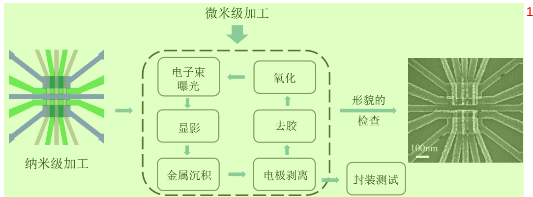
图 3.7 量子点结构的纳米级加工流程图。
