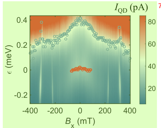
图 4.13 磁场指向面外 x 方向的漏电流随磁场大小以及双点失谐的变化。蓝色圆圈标出的为 T 态开始发生隧穿的位置。 8
