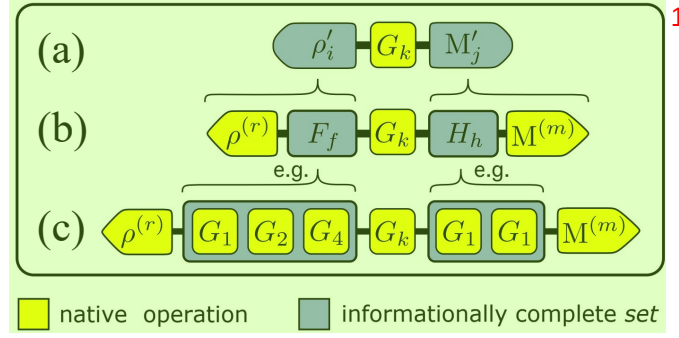
图 2.8 每个本征门 G_k 都被信息完全的有效态制备集 \rho'_i 和有效测量集 M'_j 的元素夹在中间。这些电路与处理层析测量以表征 G_k 所需的电路相同。(a) 展示了这些电路的最简单形式，每个信息完全的集合作为一个单元展示。(b) 描述有效制备（测量）集合通过在单个本征制备（测量）操作之后（之前）跟随一个基准电路 F_f ( H_h ) 来实现。(c) 举例说明基准电路是由本征门组成的，并给出了完全由本征操作表示的电路。图源自 [144] 。
