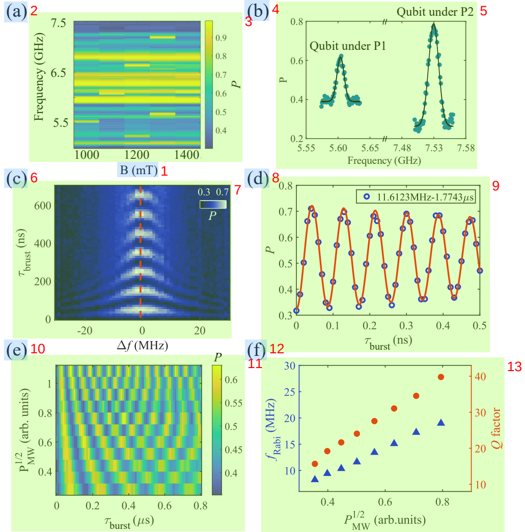
图 5.7 (a) 采用带宽为 50 MHz 的啁啾微波脉冲对量子比特共振频率进行搜索，展示了单重态概率 P 随外加微波频率及外磁场变化的二维分布。在固定磁场条件下，当微波频率与量子比特的两能级跃迁发生共振时，自旋阻塞被解除，单重态概率 P 明显增大。图中可以清晰地观察到两条具有不同斜率的共振线，分别对应两个独立量子比特的共振频率。(b) 在单频微波驱动条件下两个量子比特的共振线，分别对应各自的比特频率。(c) 单重态概率 P 随微波脉冲时长 \tau_{\text{burst}} 以及微波频率失谐变化的二维分布，呈现出典型的“V”型结构，对应量子比特的拉比振荡行为。(d) 沿 (c) 中红色虚线、即微波频率位于比特共振处时提取的拉比振荡曲线，拟合得到此处拉比频率 f_{\text{Rabi}} 为 11.61 MHz，相干时间 T_2^{\text{Rabi}} 为 1.77 \mu\text{s} 。(e) 不同微波功率下的拉比振荡结果。随着微波功率的增大，拉比振荡频率逐渐增大，表明驱动场强度增强。(f) f_{\text{Rabi}} 及品质因子 Q 随微波功率变化的关系。其中，最大 f_{\text{Rabi}} 可达 19 MHz，对应的最大品质因子 Q 为 41.10。在所测量的微波功率范围内，未观察到 f_{\text{Rabi}} 或 Q 的饱和行为。
