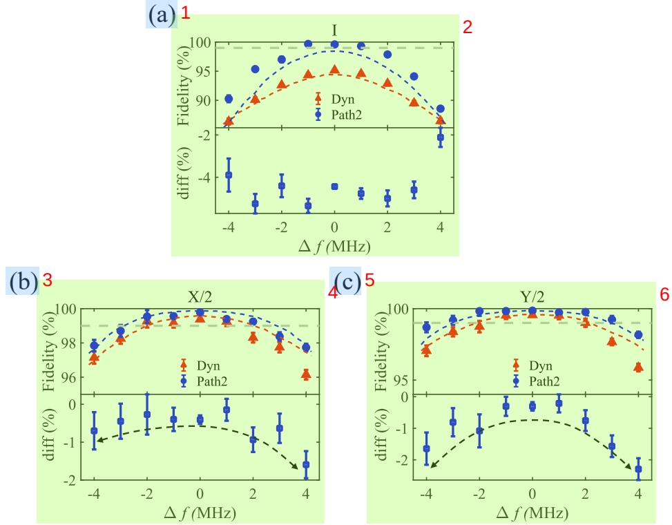
图 5.15 (a-c) 上排图展示了通过几何方式和动力学方式实现的 I 、 X/2 和 Y/2 门的控制保真度随失谐量 \Delta f 的变化关系。浅灰色实线表示 99% 控制保真度的阈值。即使当失谐量 \Delta f 达到 \pm 2.5 MHz (对于 X/2 和 Y/2 门) 或 \pm 1.2 MHz (对于 I 门) 时, 几何实现的 X/2 、 Y/2 ( I ) 门的控制保真度仍可保持在 99% 以上。下排图给出了两种实现方式之间控制保真度的差异。黑色虚线箭头作为视觉引导, 用以强调随着 \Delta f 的增大, 动力学量子门的控制保真度下降速度明显快于几何量子门。误差棒表示 95% 的置信区间。实验结果与数值模拟结果 (蓝色和红色虚线) 一致。
