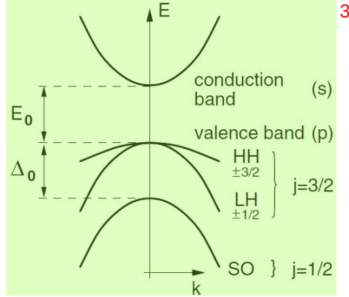
图 4.6 自旋-轨道相互作用导致最上方价带发生分裂, 劈裂的能量差为 \Delta_0 。由于应力或者缺陷的影响, j = 3/2 的价带会进一步劈裂成为重空穴带与轻空穴带。图源自 [225]。
