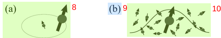
图 4.2 (a) 一个电子自旋与 (a) 原子中的单个核自旋相互作用，与 (b) 半导体量子点中的多个核自旋相互作用。图源自 [109] 。 11
