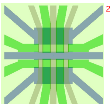
图 3.4 量子点结构最中心百纳米范围内的设计图。
