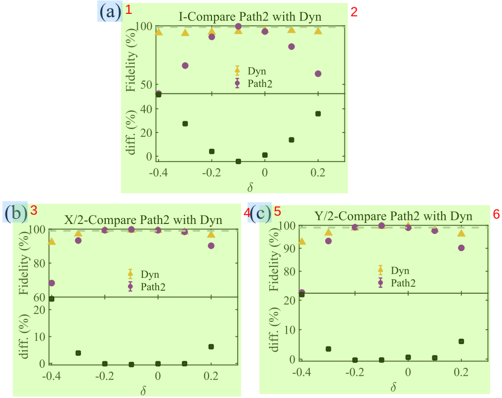
图 5.19 (a-c) 添加拉比频率抖动噪声 \delta 的情况下 Path2 几何量子门与传统动力学的保真度对比，发现针对于比特频率抖动噪声 \Delta f 设计的几何门 Path2 对于 \delta 基本没有抗性。误差棒代表 95% 置信水平。
