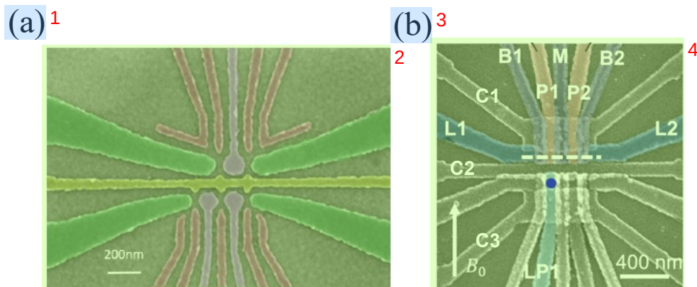
图 3.3 (a) 单层电极量子点结构。(b) 重叠栅极量子点结构。
