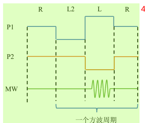
图 3.15 方波脉冲、微波操控信号及各触发信号之间的相对时间关系示意图。 5
