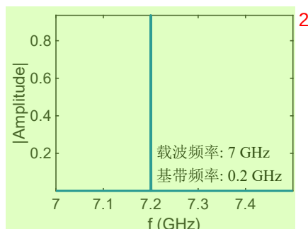
图 3.16 IQ 混频校准之后的微波频谱情况。
