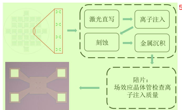
图 3.6 量子点微米级加工流程图示意图。 6
