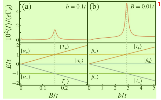
图 4.4 (a) 施加面内磁场时, 双量子点 g 因子差异引起的漏电流随外磁场的变化。下方为能级示意图, 当三重态 |T_{\pm}\rangle 与 S(1, 1) 和 S(2, 0) 的叠加态 |\alpha_{\pm}\rangle 发生共振时, 对应磁场下出现电流峰。(b) 施加面外磁场时, 双量子点 g 因子差异引起的漏电流随外磁场的变化。当三重态 |T_{\pm}\rangle 与 S(1, 1) 和 S(2, 0) 的叠加态 |\beta_{\pm}\rangle 发生共振时, 对应磁场下出现电流峰图源自 [168] 。
