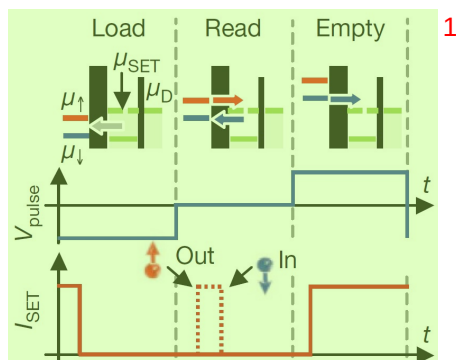
图 2.2 自旋选择隧穿读取的原理示意图。此处的载流子为电子。当量子点中存在电子占据时，对应电荷探测器的响应信号为零，无电子占据时，电荷探测器会产生非零电流响应。当量子点中存在一自旋向上的电子，在读取（Read）阶段自旋向上的电子可以跳出，随即一自旋向下的电子跳入。单发读取的信号在 Read 阶段出现一个信号峰值。图源自 [116]。
