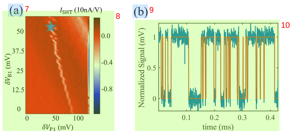
图 3.13 (a) 量子点与源漏的隧穿速率可调，随着 B1 电压的逐渐变大，量子点的隧穿信号从聚集而清晰变得分散而微弱，说明量子点与源漏之间的隧穿速率从大变小的过程。(b) 量子点的随机电报信号，归一化信号在 0 到 1 之间变化，说明空穴在隧穿线处的随机隧穿过程。
