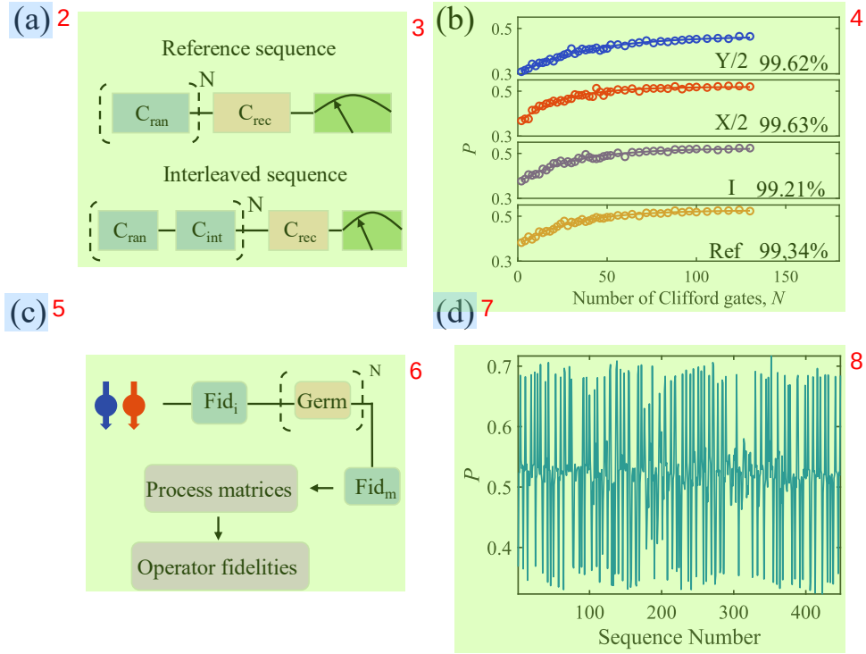
图 5.9 (a) 随机基准序列实验的序列示意图，上半部分为参考序列，下半部分为插入门实验。(b) 随机基准序列实验的结果，包括 Clifford 门以及 X/2 、 Y/2 和 I 门的保真度结果。它们的操控度均超过了容错量子计算的阈值 (c) 门集层析测量量子比特操控保真度的序列示意图 (d) 采用线路深度 L = 8 的门集层析 (GST) 序列，共 448 个序列的输出结果。
