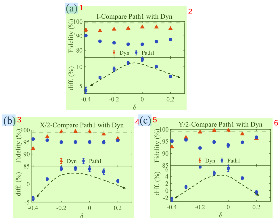
图 5.17 (a-c) 上半部分展示了在不同 \delta 噪声条件下量子门操控保真度的变化情况，下半部分为几何门 Path1 与传统动力学门操控保真度的差值。
