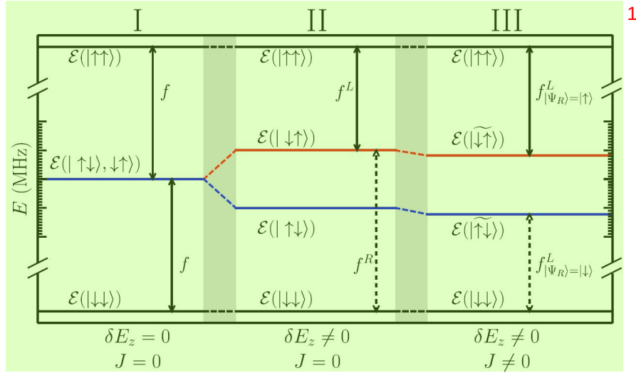
图 2.5 两个自旋在存在磁场梯度的双量子点中的本征能量 E ，以及在三种不同参数区域下它们之间的相关跃迁。区域 I 描述的是没有磁场梯度的情况，此时单自旋翻转跃迁在能量上是简并的。区域 II 表示在存在磁场梯度时，左侧自旋与右侧自旋之间的跃迁频率简并被打破，从而可以从能量上区分对左自旋和右自旋的单比特操作。进一步打开交换相互作用 J （区域 III），左侧自旋的共振频率会依赖于右侧自旋的状态，因此可以通过频率选择实现两比特门操作。图源自 [137] 。
