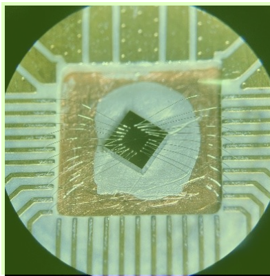
图 3.8 用银胶贴片在 PCB 板上的量子点芯片，芯片引脚与 PCB 板通过铝线键合。 4
